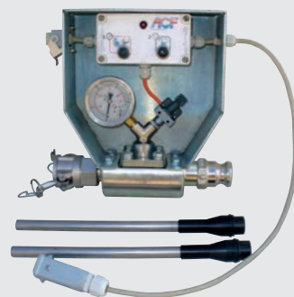
Kit "Speciale iniezione" P 737
