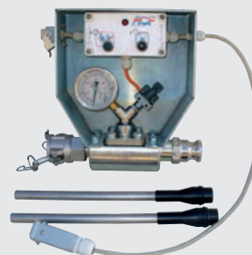
Kit "speciale Iniezione" P 731
